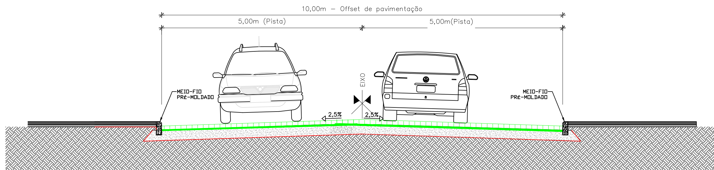
SEÇÃO TIPO DE PAVIMENTAÇÃO- Offset de pavimentação com bloco intertravado-RUA CARLOS AUGUSTO BERLT
